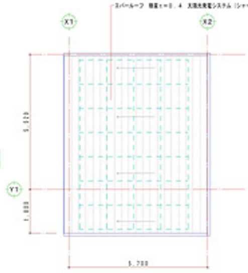
屋根平面図 S=1:100
